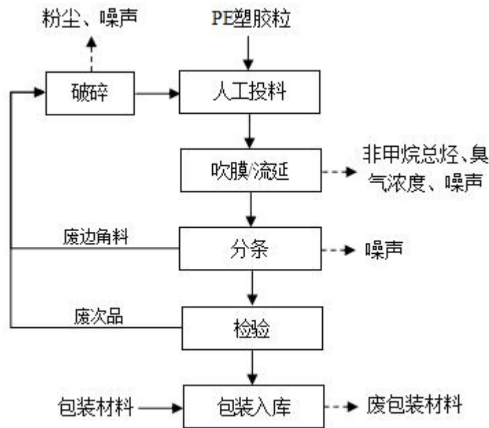
图 2-2 项目包装膜生产工艺流程图
