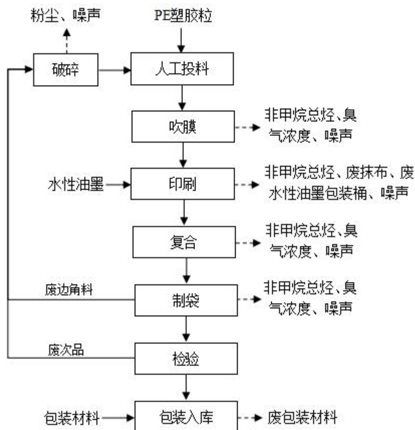
图 2-3 项目包装袋生产工艺流程图
