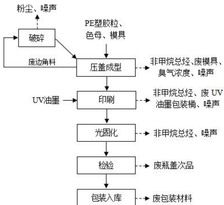
图 2-3 项目 PE 瓶盖生产工艺流程图
