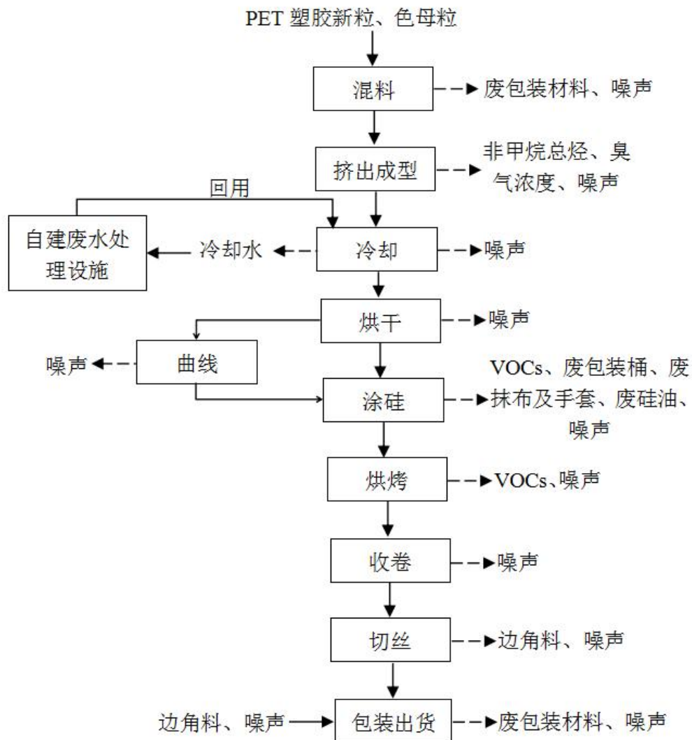
图 2-2 项目生产工艺流程
