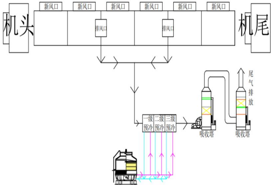
图 4.1-1 NMP 冷凝回收处理系统工艺流程图
