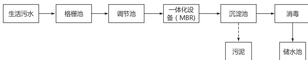
图 4.2-1 项目自建生活污水处理站工艺图
