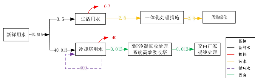
图2.7-1 近期项目水平衡图 (t/d)
