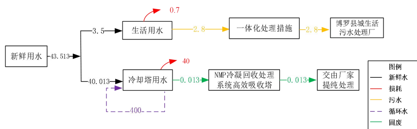
图2.7-2 远期项目水平衡图 (t/d)
