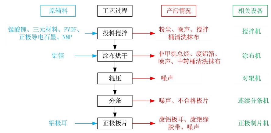
图2.11-1 正极制片工艺流程图
