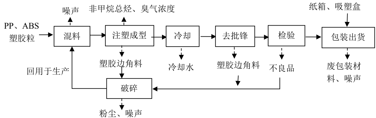
图 2-2 项目电动车配套塑胶件生产工艺流程图
