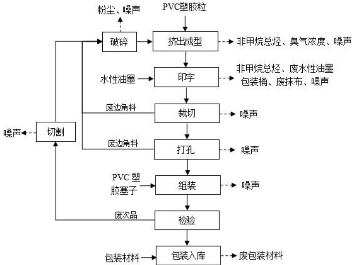
图 2-3 项目 PVC 方管生产工艺流程图
