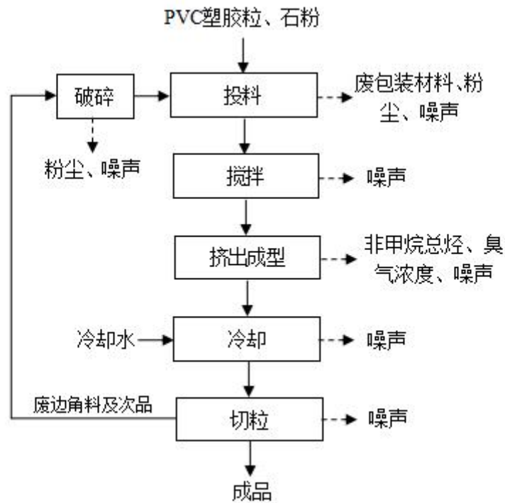
图 2-2 项目 PVC 改性塑胶粒生产工艺流程图
