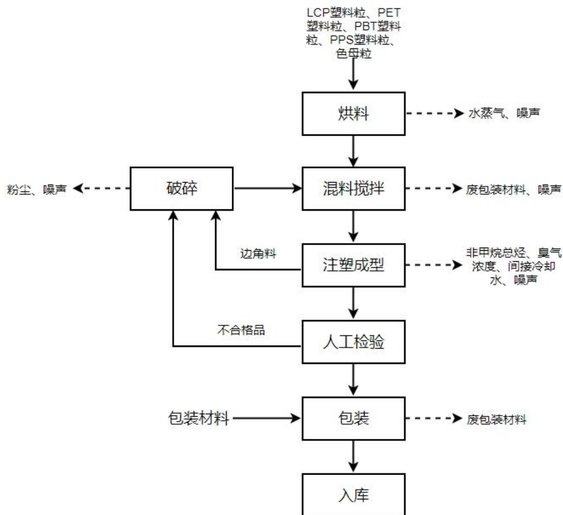
图2-3 项目塑胶外壳生产工艺流程图
