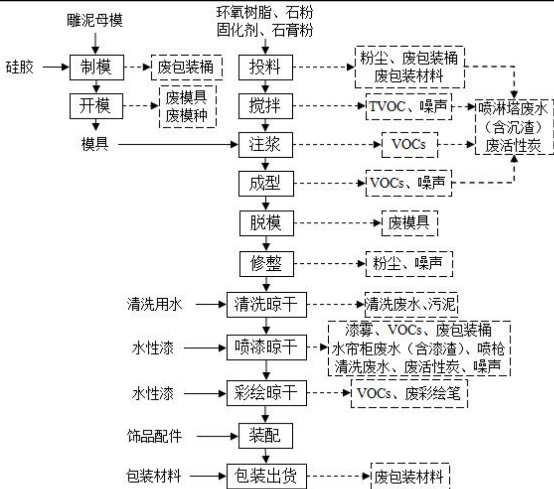
图 2-4 项目工艺流程及产污环节图
