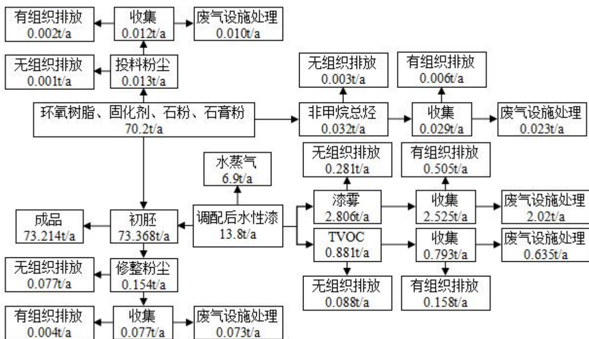
图 2-3 项目物料平衡图
