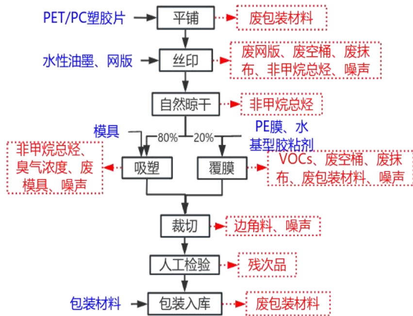
图 2-3 项目丝印塑胶片生产工艺流程图
