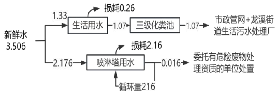
图 2-2 项目水平衡图 (t/d)
