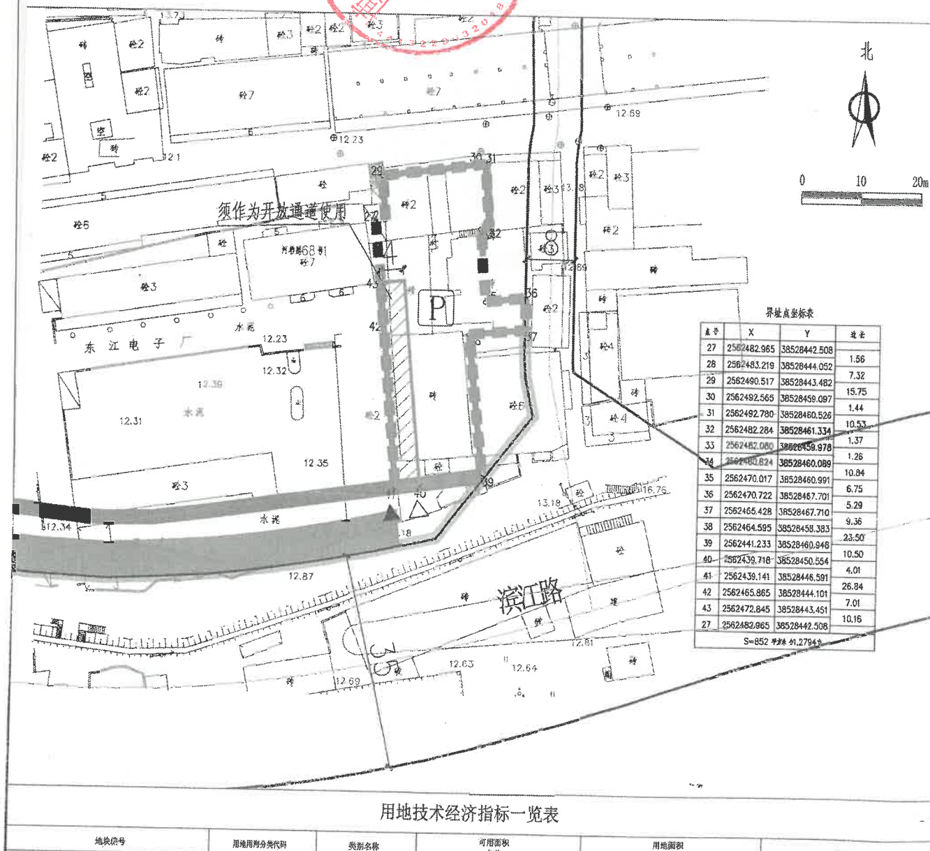
博罗县2024（储备）24号用地规划设计要点图
