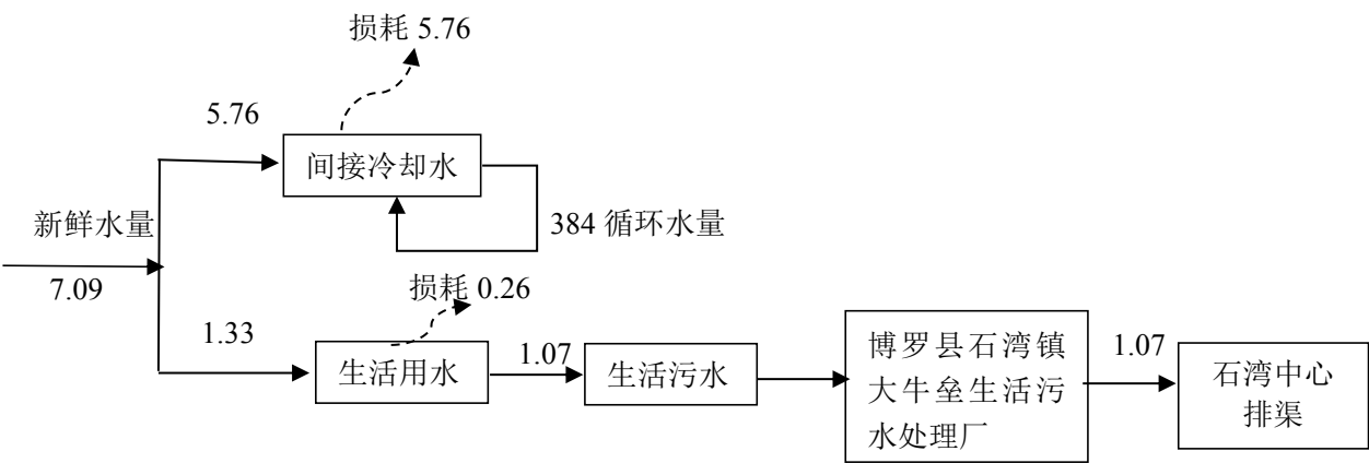
图 2-1 项目水平衡图（m³/d）
