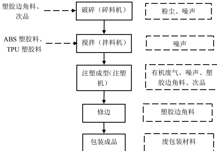
图 2-3 原项目原手机套、手机支架生产工艺流程图
