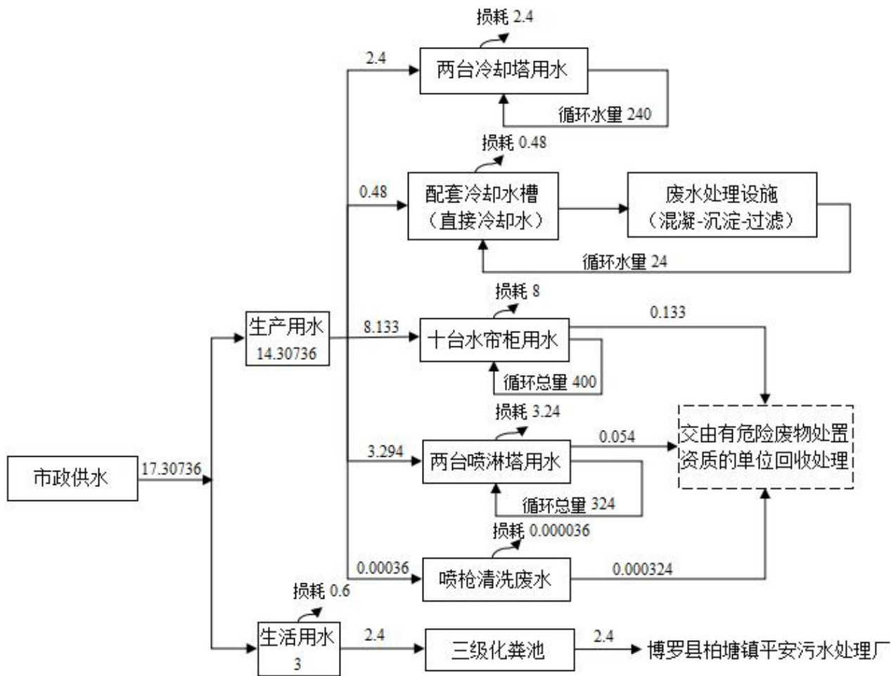
图 2-1 项目水平衡图 (t/d)
