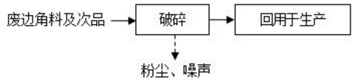
图 2-3 项目废边角料及次品回用工艺流程及产污环节图
