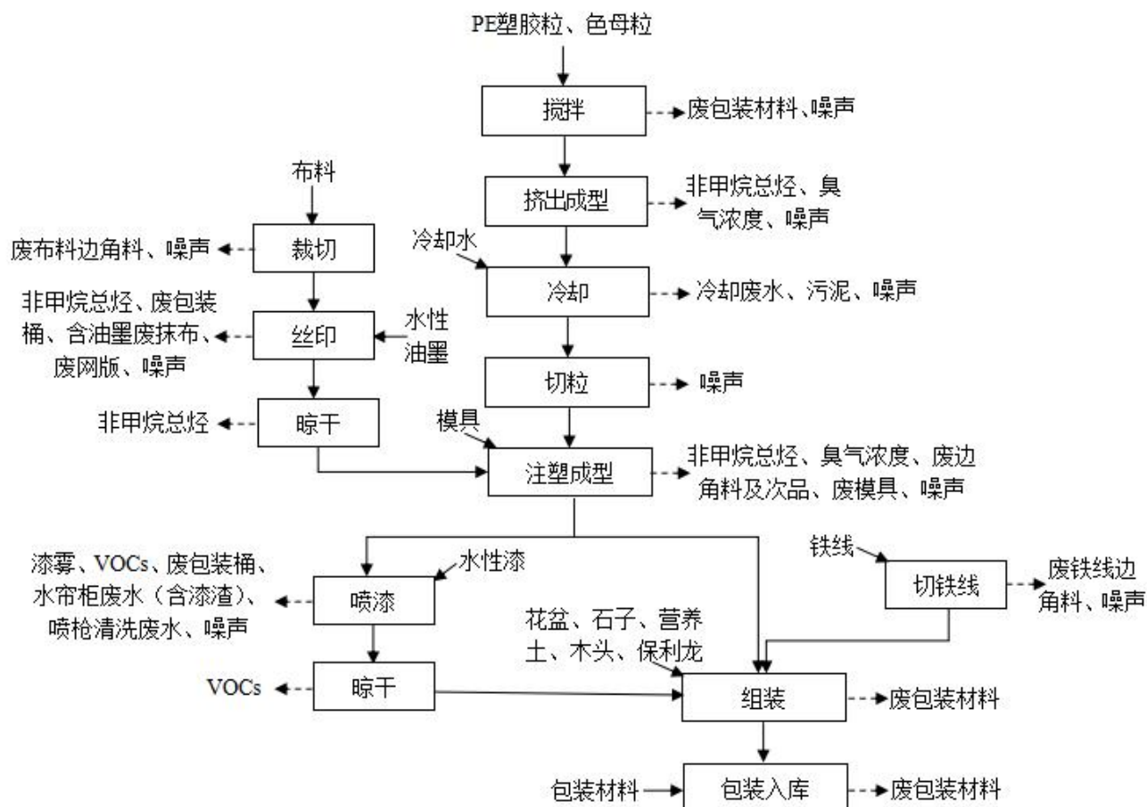
图 2-2 项目工艺流程及产污环节图
