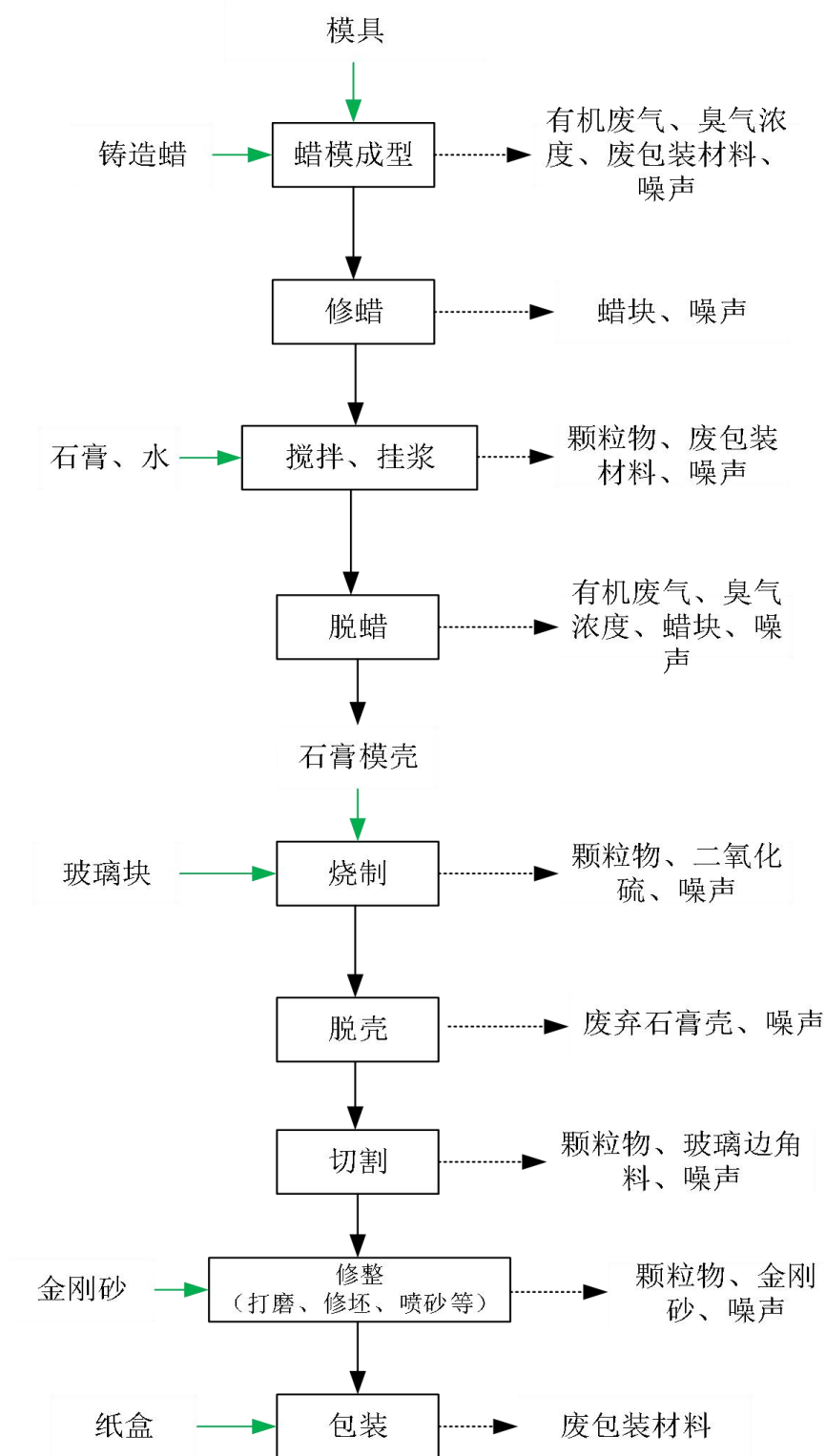
图2-2产品生产工艺流程图
