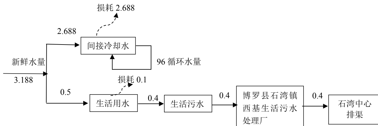
图 2-1 项目水平衡图（m 3 /d）
