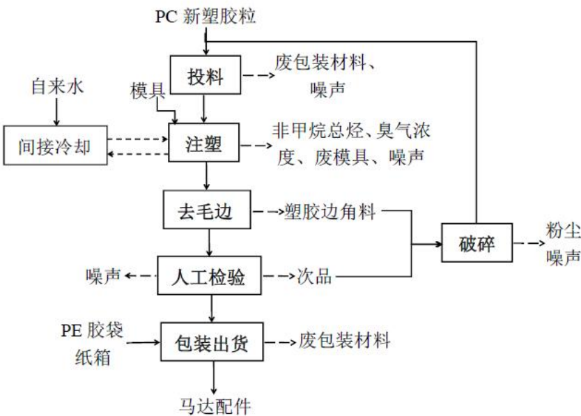
图 2-3 项目马达配件生产工艺流程
