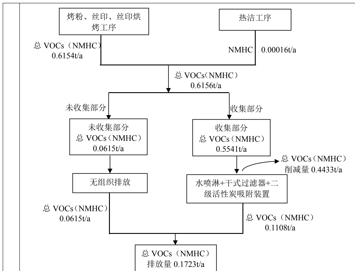
图 4 项目总 VOCs (NMHC) 物料平衡图
