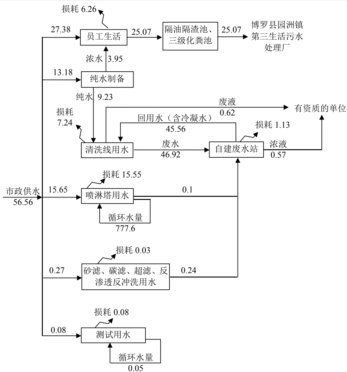
图 3 项目水平衡图（远期） 单位： \text{m}^3/\text{d}
