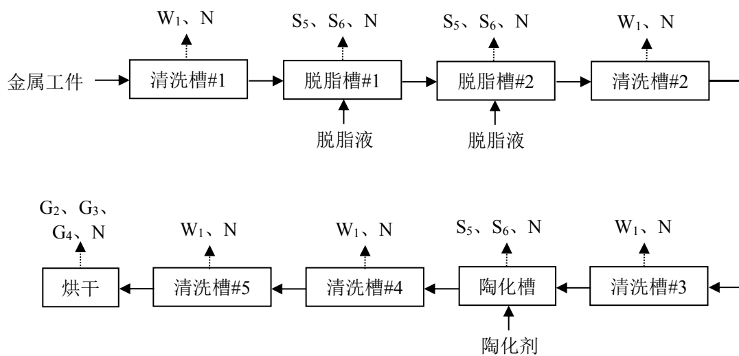
图 7 自动清洗线生产工艺示意图
