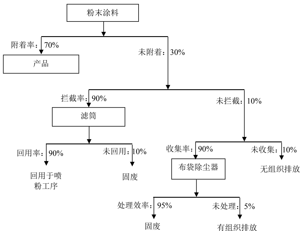
图 1 喷粉工序粉末涂料利用情况示意图
