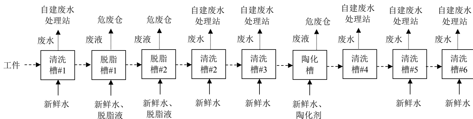
图 14 手动清洗线各槽体连接情况示意图
