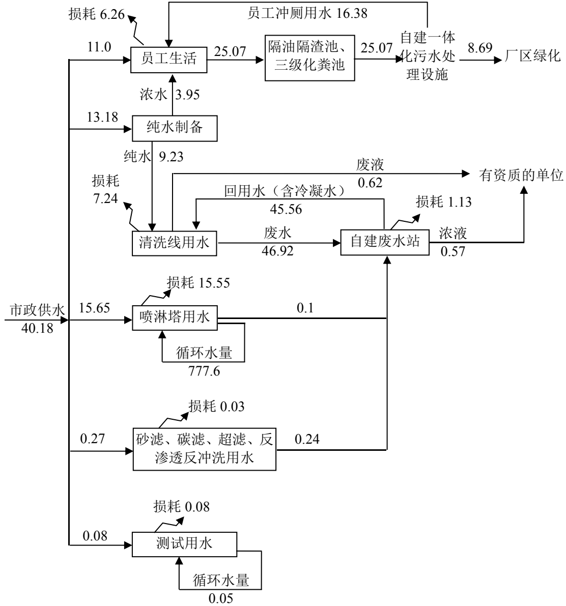
图 2 项目水平衡图 (近期) 单位: \text{m}^3/\text{d}
