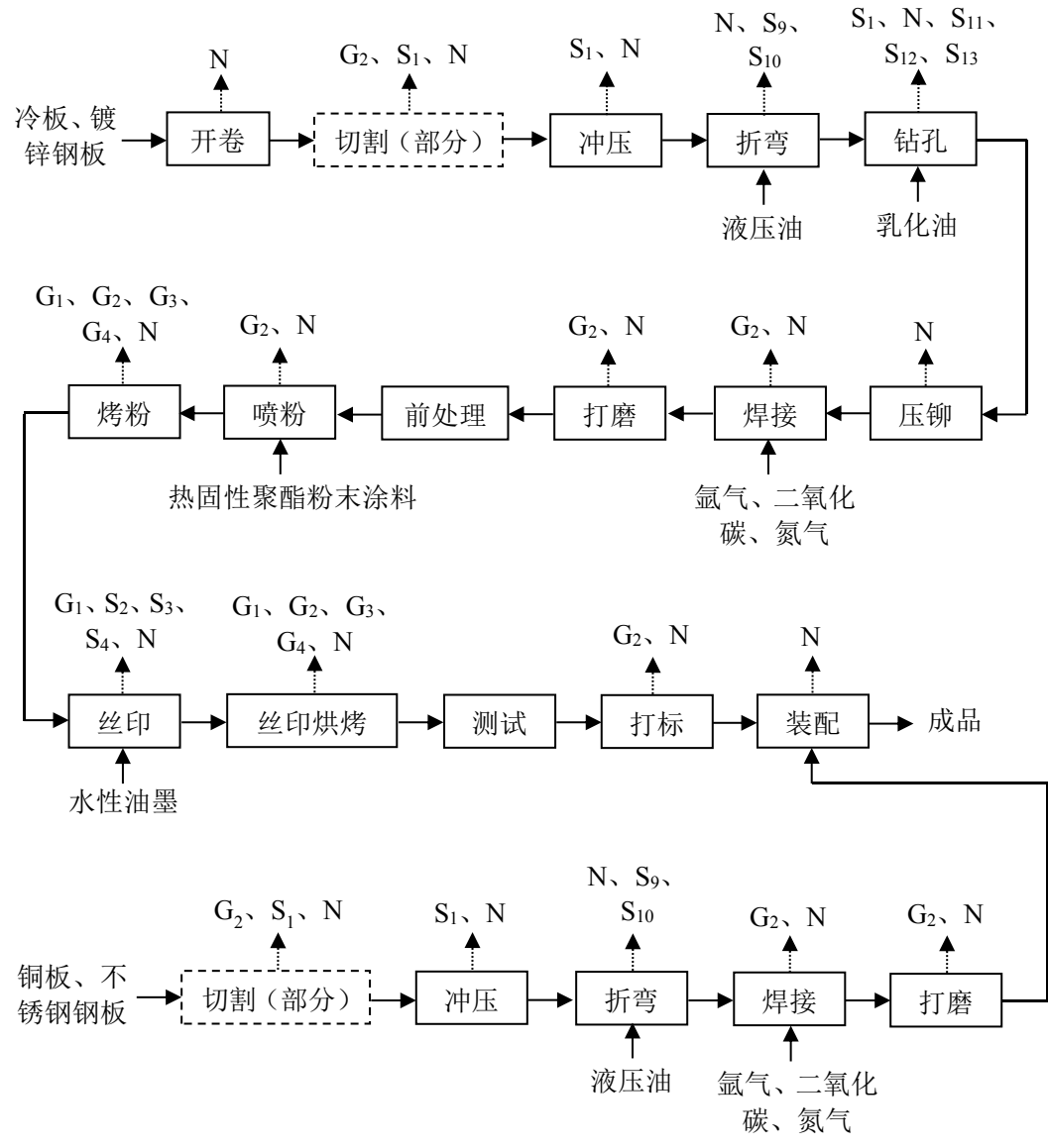
图 5 项目智能 IT 服务器机柜体、智能 5G 通信基站电源系统柜体、智能 UPS 电源系统柜体、电源插框生产工艺示意图
