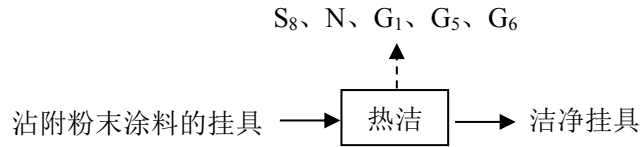
图 10 项目热洁工艺及产污环节示意图
