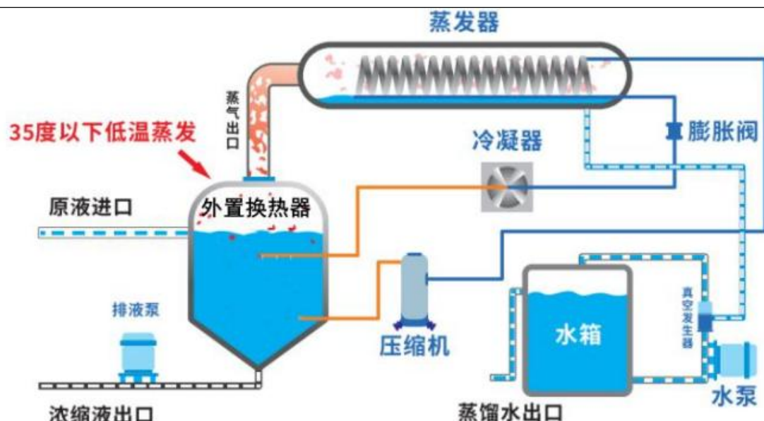
图 17 低温蒸发器示意图
