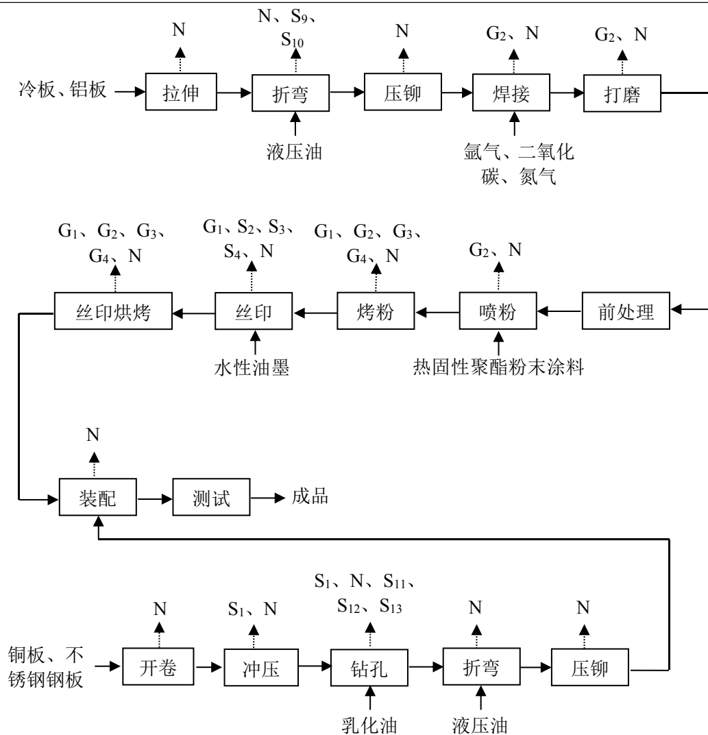
图 6 项目逆变器柜体生产工艺示意图
