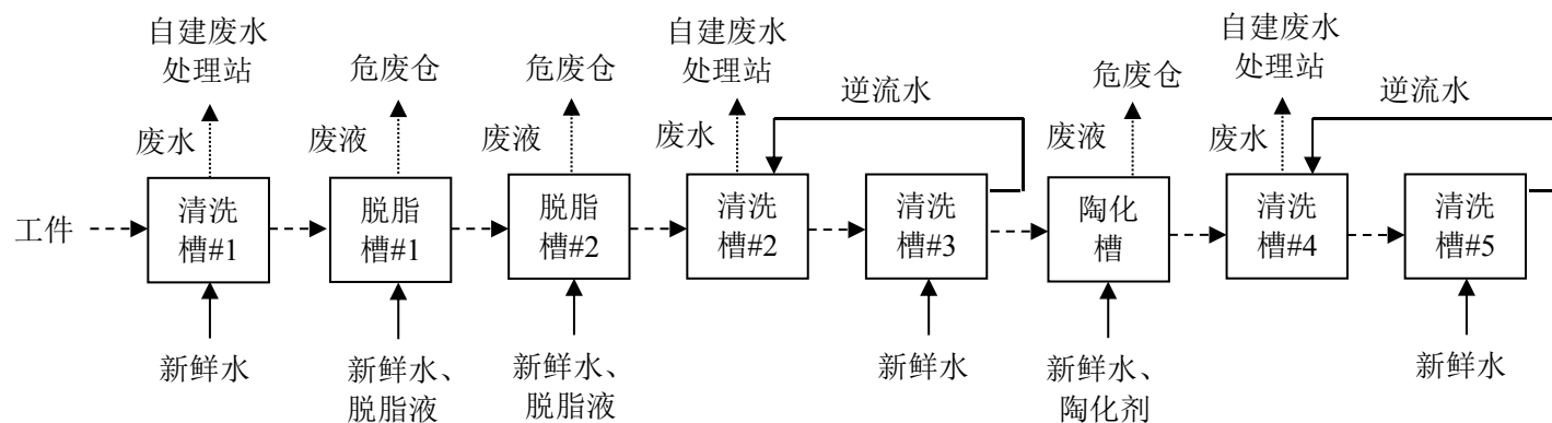
图 15 自动清洗线各槽体连接情况示意图
