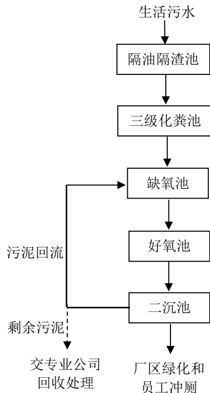
图 18 项目生活污水处理工艺流程图
