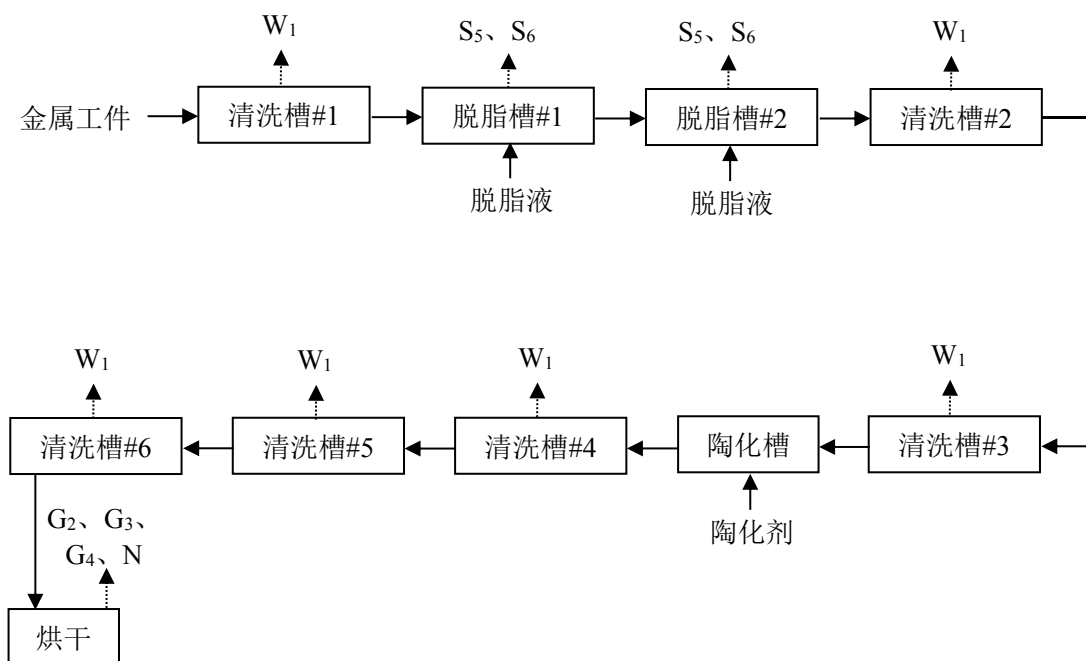
图 8 手动清洗线生产工艺示意图
