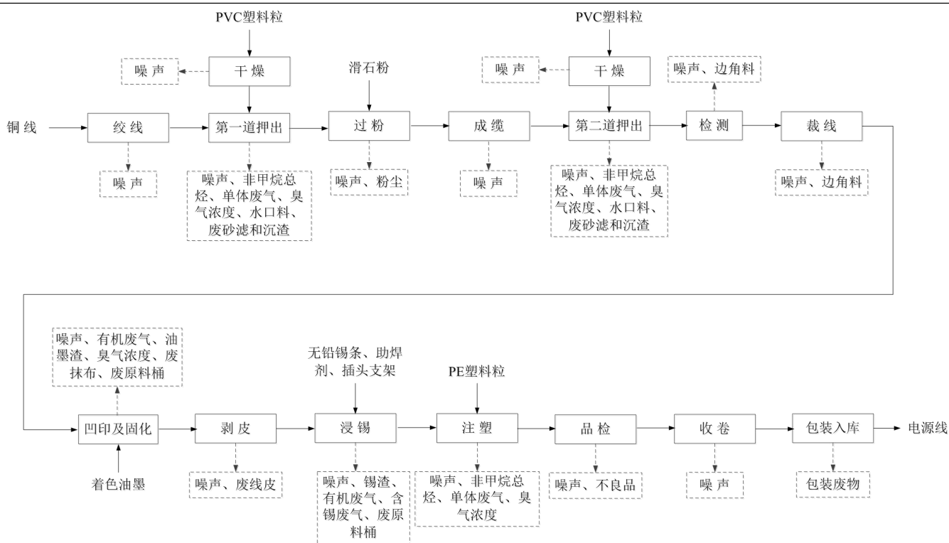
图3 项目电源线生产工艺流程及产污环节图
