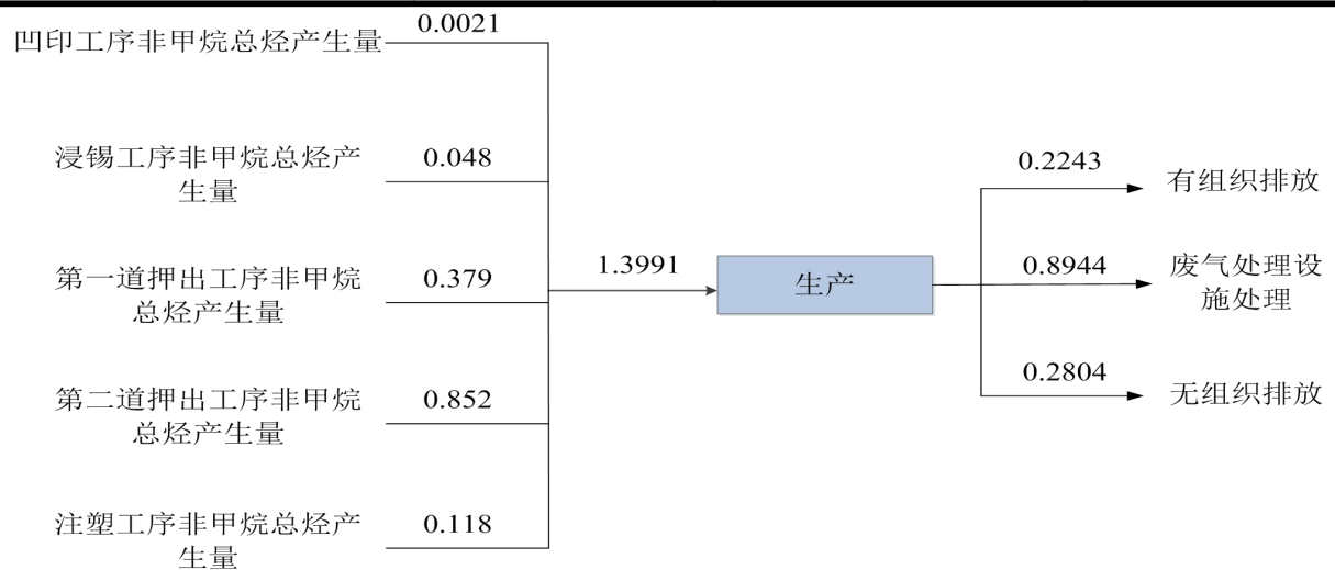
图 2 项目 VOCs 平衡图 (单位: t/a)
