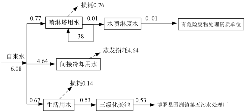
图 1 项目水平衡图 单位: t/d
