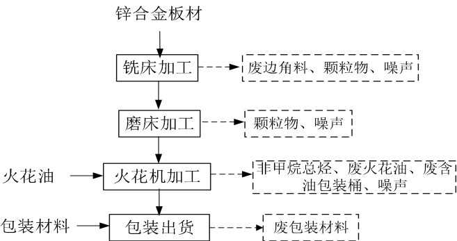
图3 模具生产工艺流程图及产污环节
