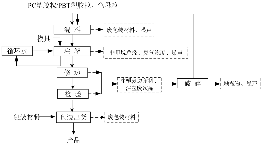
图 2 散热风扇塑胶件生产工艺流程图及产污环节
