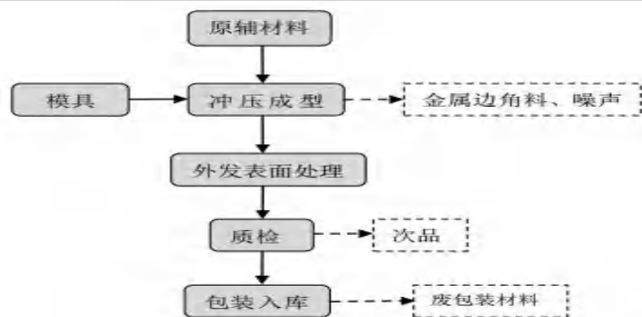
图3 项目外壳、支架、端子、刷子、弹片生产工艺流程图及产污节点图
