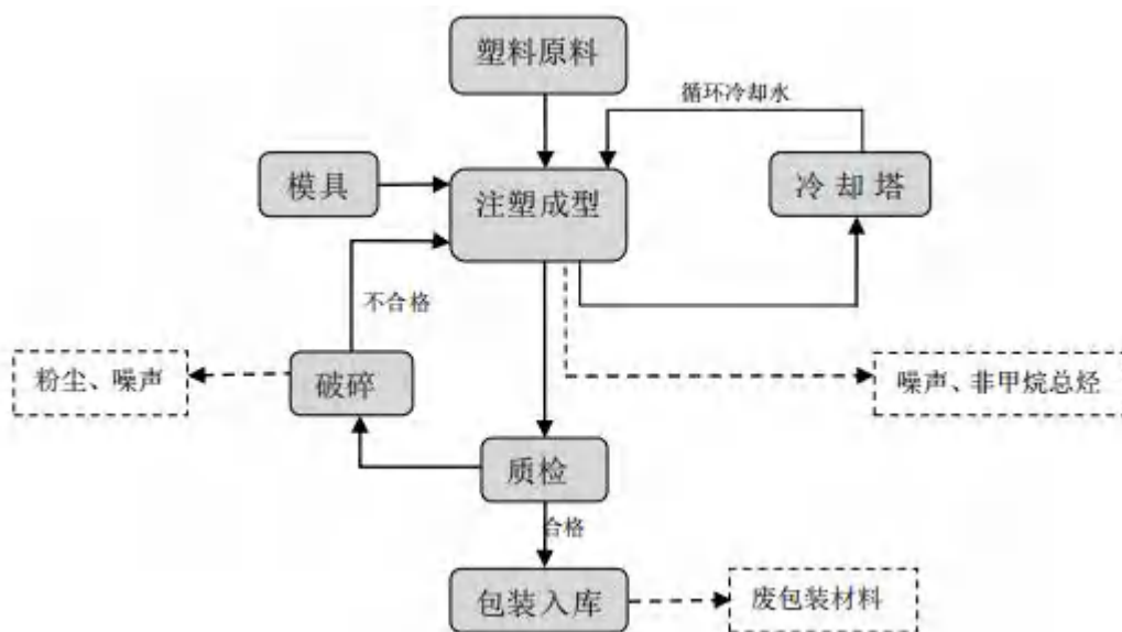
图2 项目塑料制品生产工艺流程图及产污节点图
