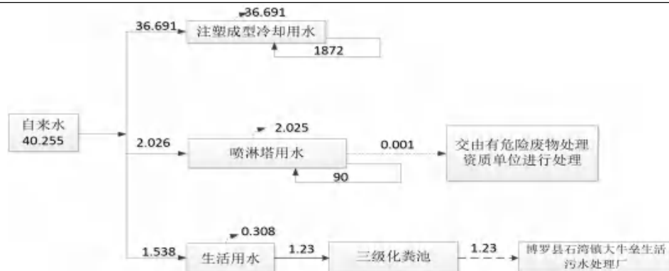
图1 迁改扩建项目水平衡图 单位: t/d
