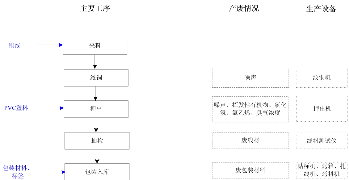
图 2-3 线材生产工艺流程及产排污节点图 2
