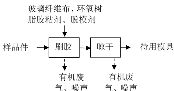
图 2-6 自制模具（机身模具、机翼模具）生产工艺流程图
