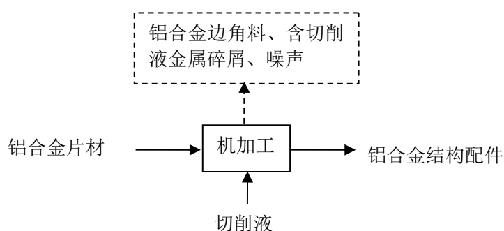
图 2-3 无人机-铝合金结构配件部分的生产工艺流程图
