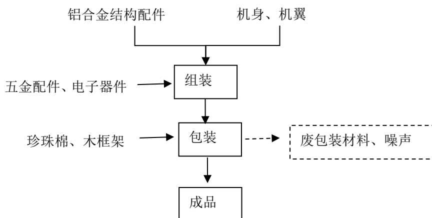
图 2-4 无人机-组装部分的生产工艺流程图
