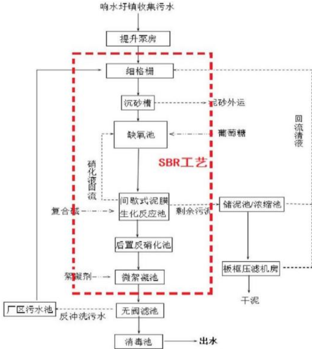
图 4-1 博罗县湖镇镇响水埔头生活污水处理厂工艺流程图
