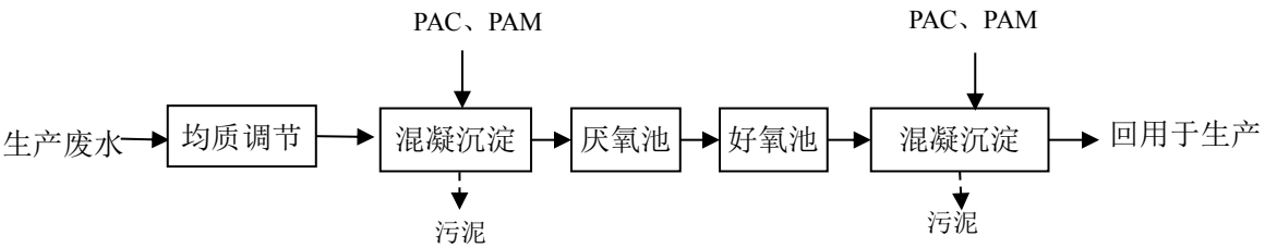
图 6 废水处理工艺流程图
