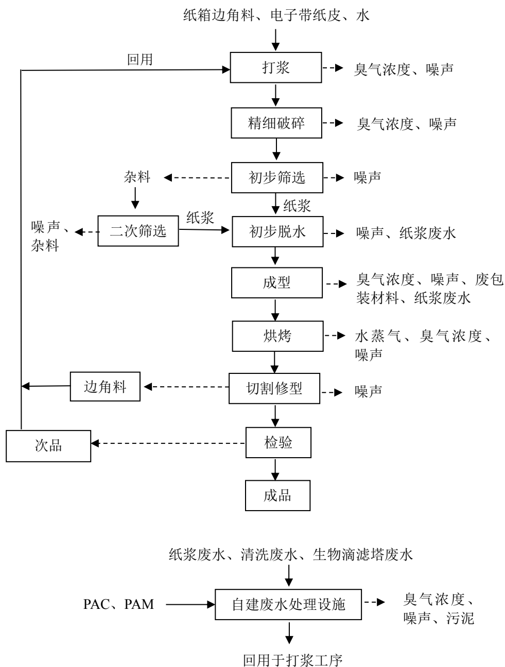
图2 纸托生产工艺流程图示意图
