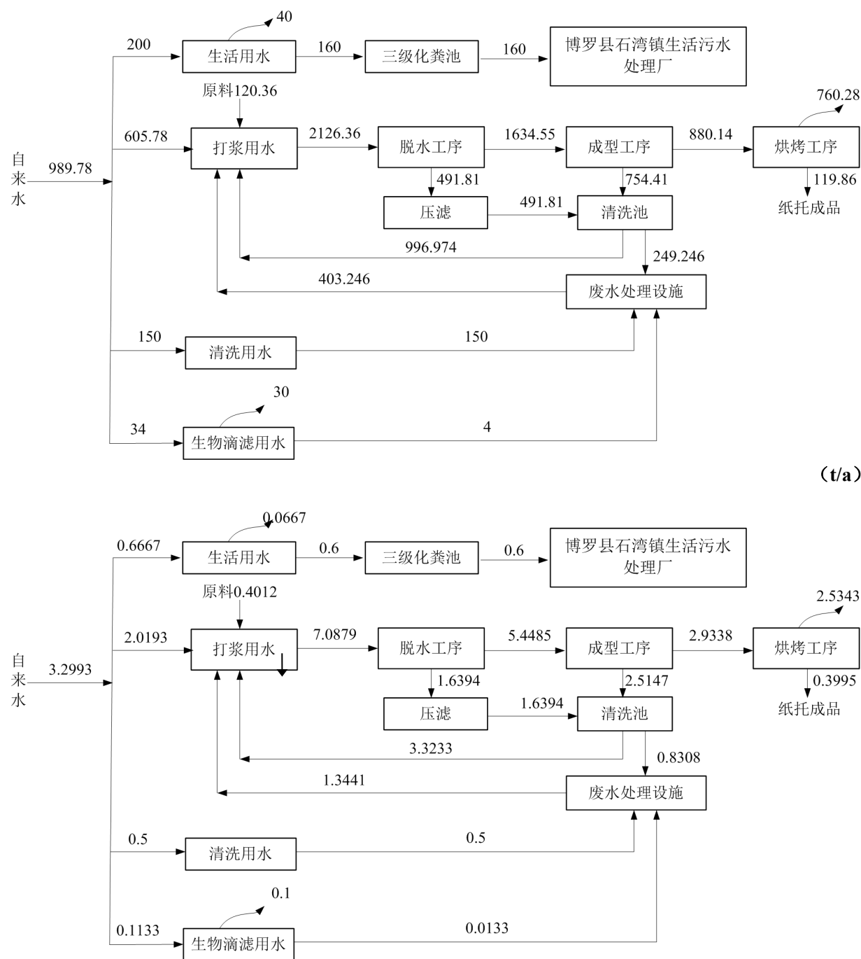
图 1 水平衡图 (t/d)
