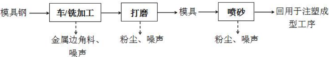
图 2-3 项目模具生产工艺
