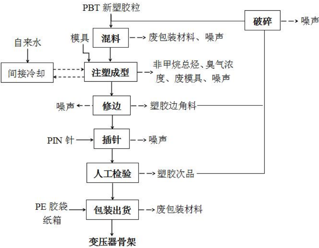
图 2-2 项目变压器骨架生产工艺流程
