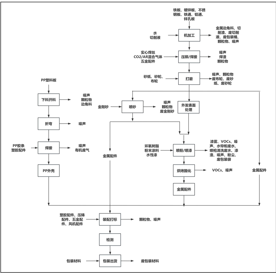
图 2-4 项目风机生产工艺流程图
