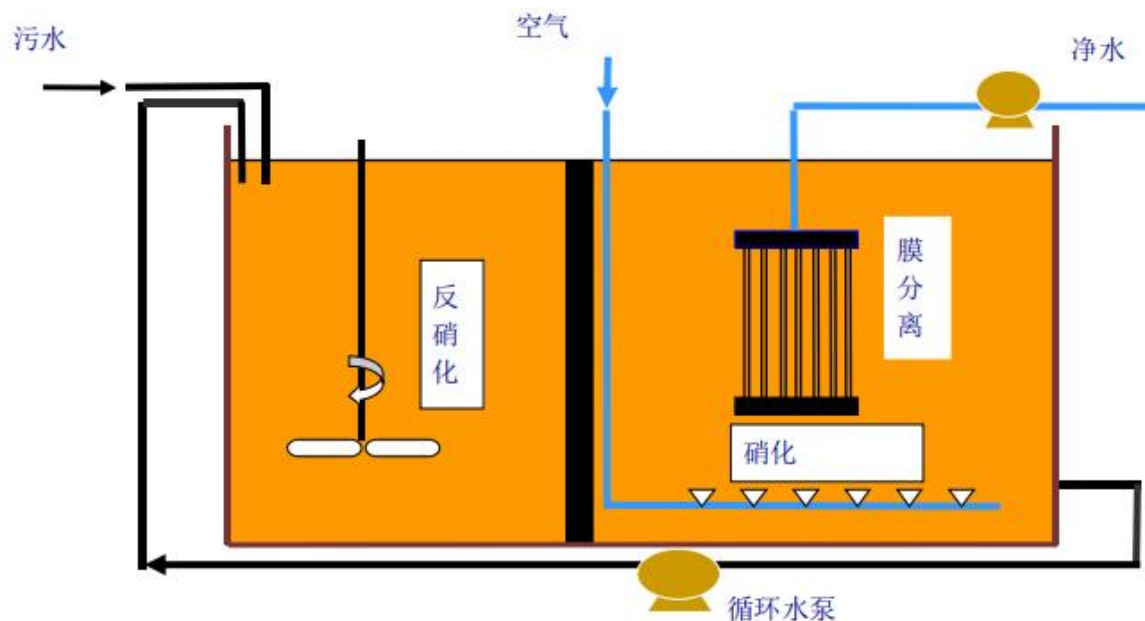
图 4-4 MBR 反应器示意图
