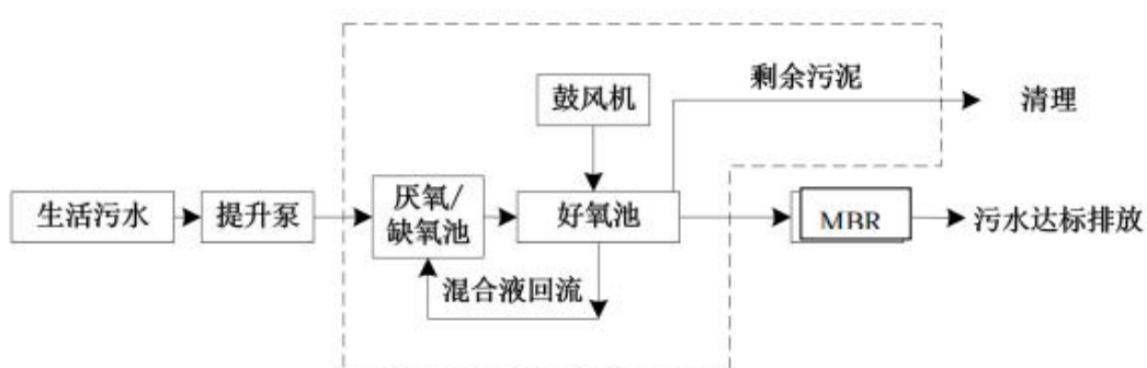
图 4-2 自建生活污水处理设施处理工艺流程
