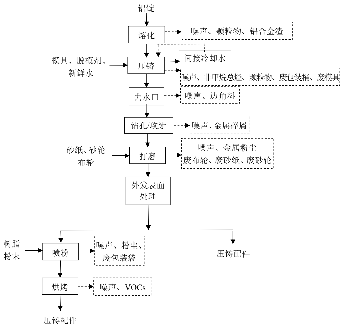
图 2-2 项目压铸铝合金配件生产工艺流程图
