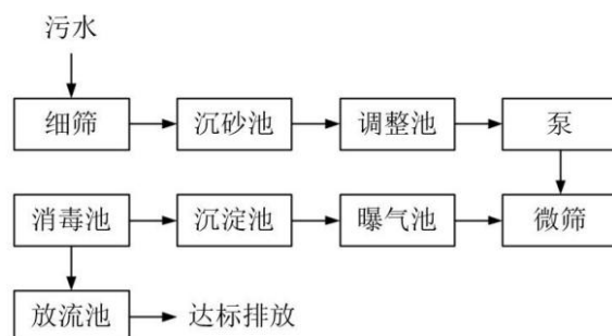
图 4-1 污水处理厂处理工艺流程
