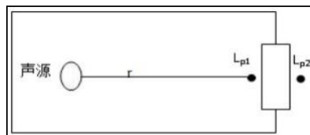
图 4-5 室内声源等效为室外声源图例
