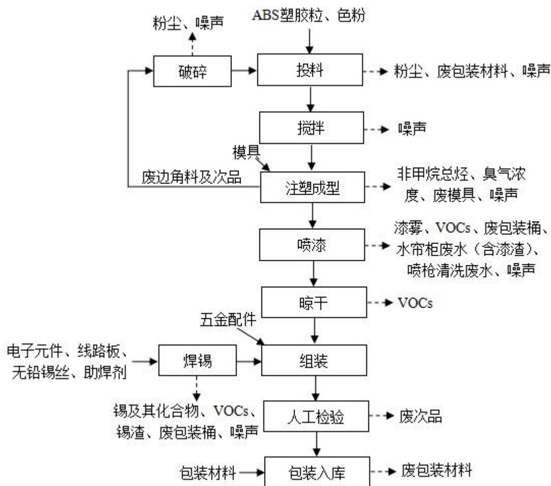
图 2-2 项目工艺流程及产污环节图
