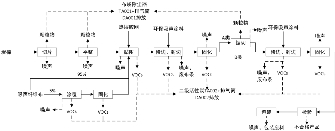
图 2-2 岩棉天花板生产工艺流程图
