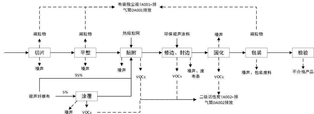
图 2-3 岩棉墙板生产工艺流程图
