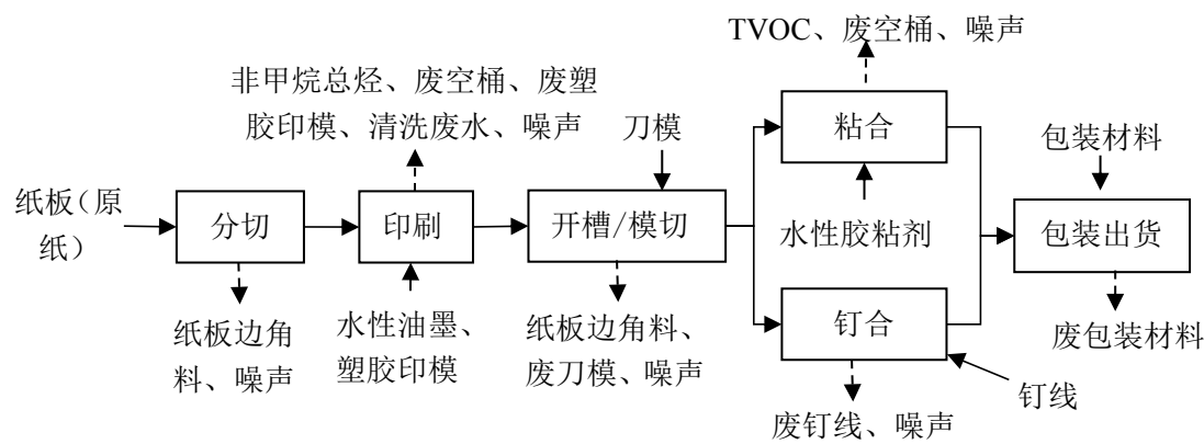
图 2-2 项目纸箱产品生产工艺流程图
