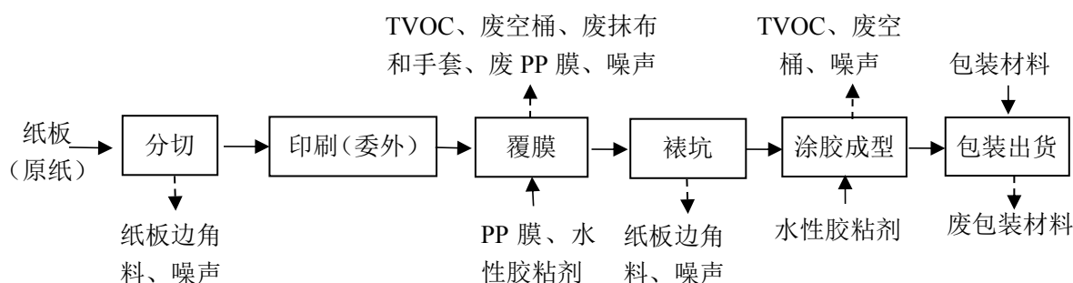
图 2-3 彩盒生产工艺流程图
