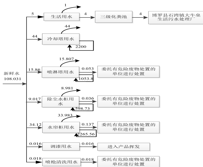
图 1 项目水平衡图（t/d）
