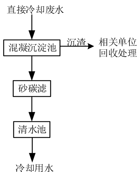
图 4-3 废水处理工艺图
