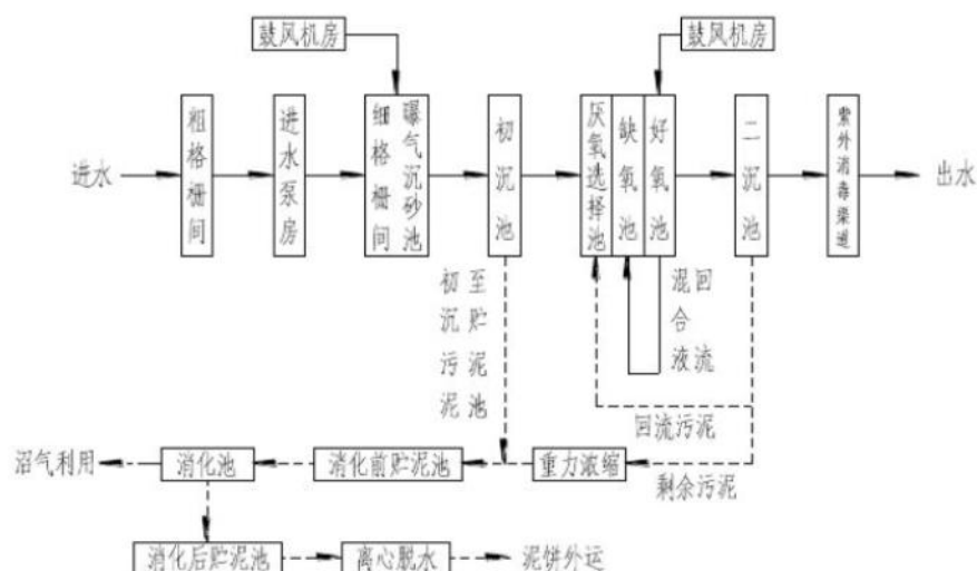
图 4-2 博罗县龙溪街道生活污水处理厂工艺流程图
