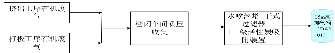
图 4-1 项目有机废气处理工艺流程图
