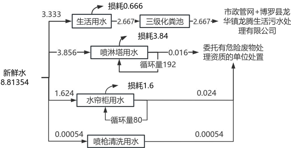
图 2-3 迁改扩建项目水平衡图 (t/d)
