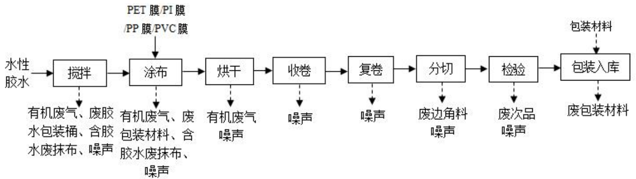
图 2-2 项目生产工艺流程及产污环节图
