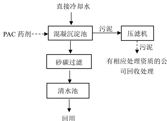
图 4-1 废水处理工艺
