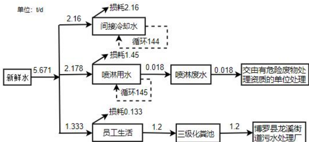
图 2-2 改扩建后全厂水平衡图（单位：t/d）
