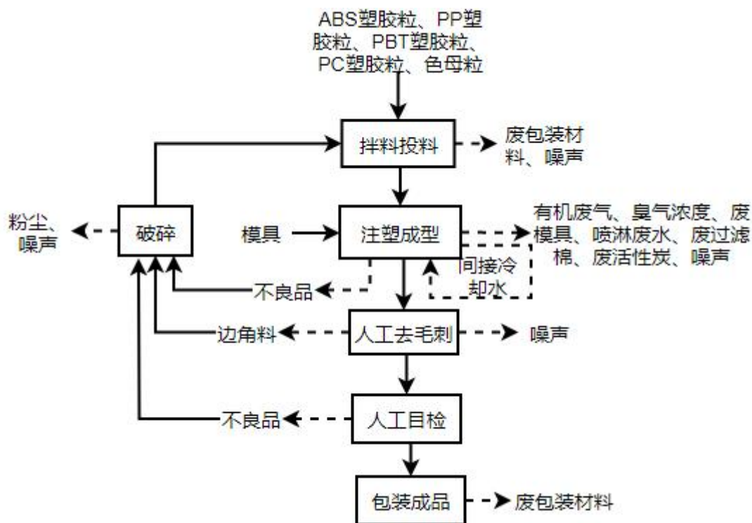
图 2-3 改扩建项目生产工艺流程图
