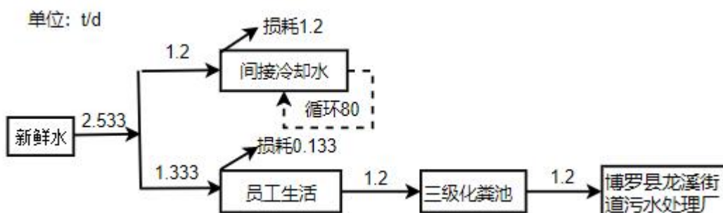
图 2-1 现有项目水平衡图（单位：t/d）
