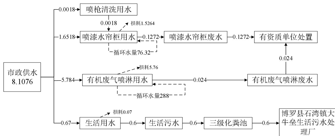
图 2-1 项目水平衡图 (单位: \text{m}^3/\text{d} )
