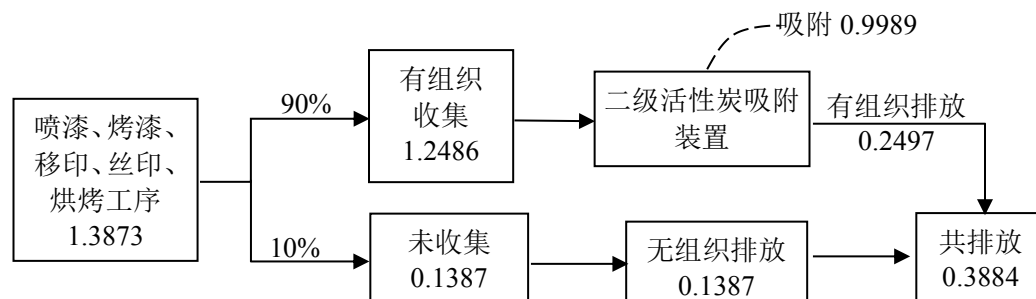
图 2-2 项目挥发性有机物平衡图 ( \text{t/a} )
