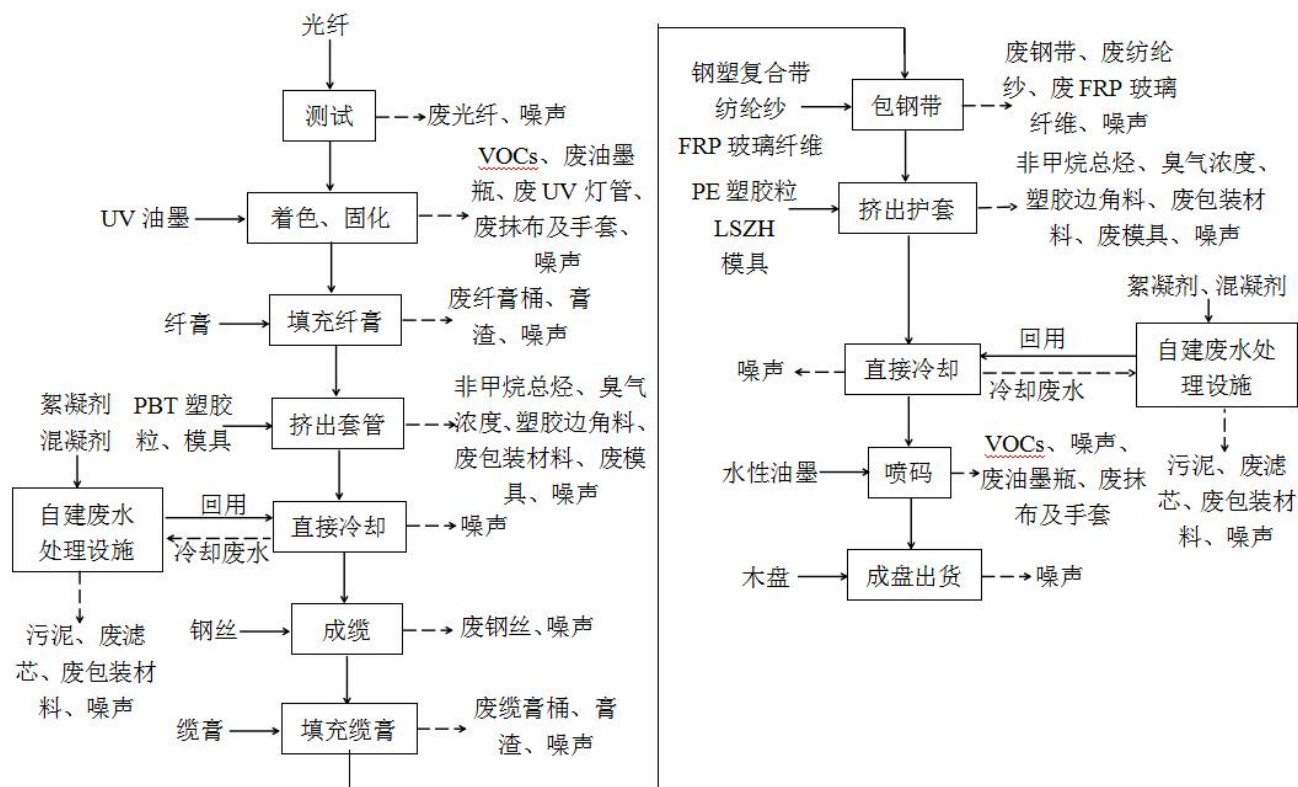
图 2-2 项目室外通信光缆生产工艺流程
