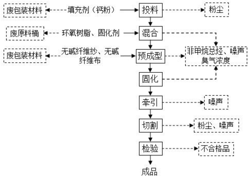
图 2-3 项目玻璃钢拉挤管工艺流程及产污环节图
