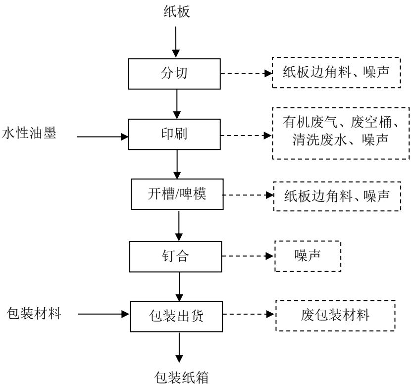
图 2-3 包装纸箱生产工艺流程及产污环节示意图
