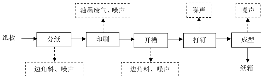
图 2-5 包装纸箱生产工艺流程及产污环节示意图
