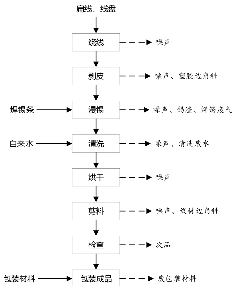
图 2-2 线圈（扁线类）生产工艺流程图
