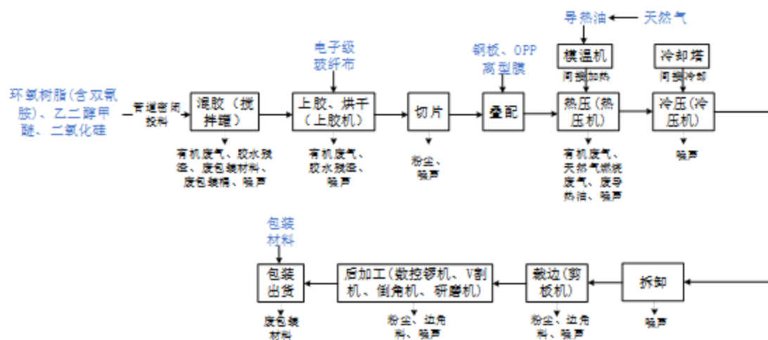
图 2-2 项目环氧绝缘板生产工艺流程图
