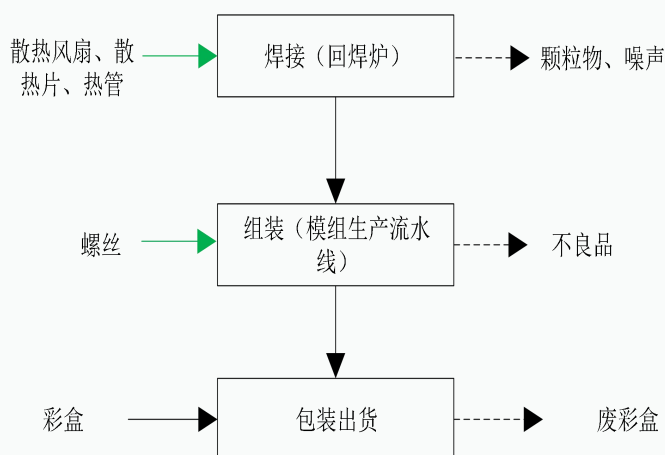
图 2-4 项目散热模组生产工艺流程图
