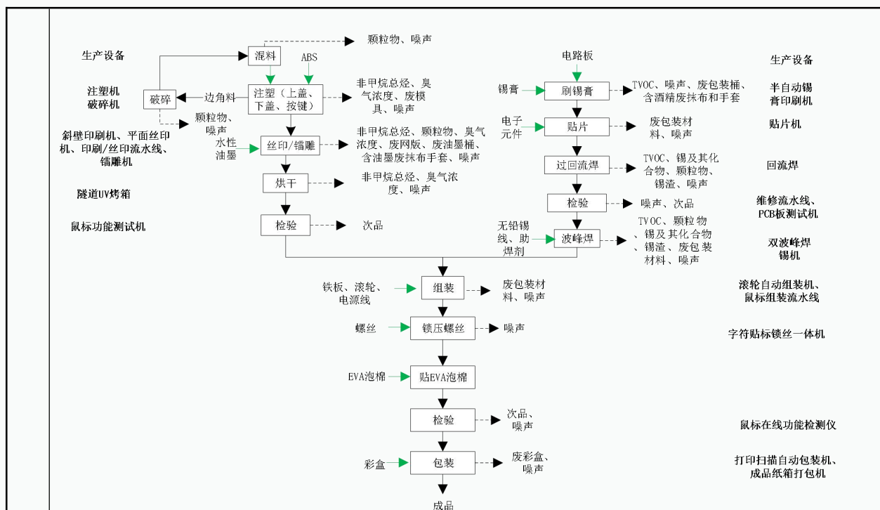
图2-2项目鼠标生产工艺流程图
