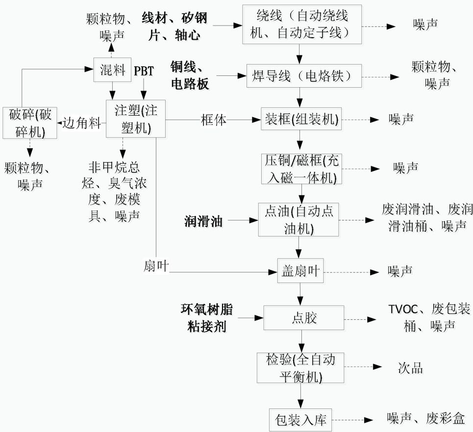
图 2-3 项目散热风扇生产工艺流程图
