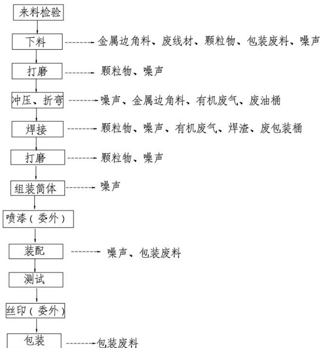
图 2-11 吸附式干燥机、制氧机、制氮机工艺流程及产污环节示意图
