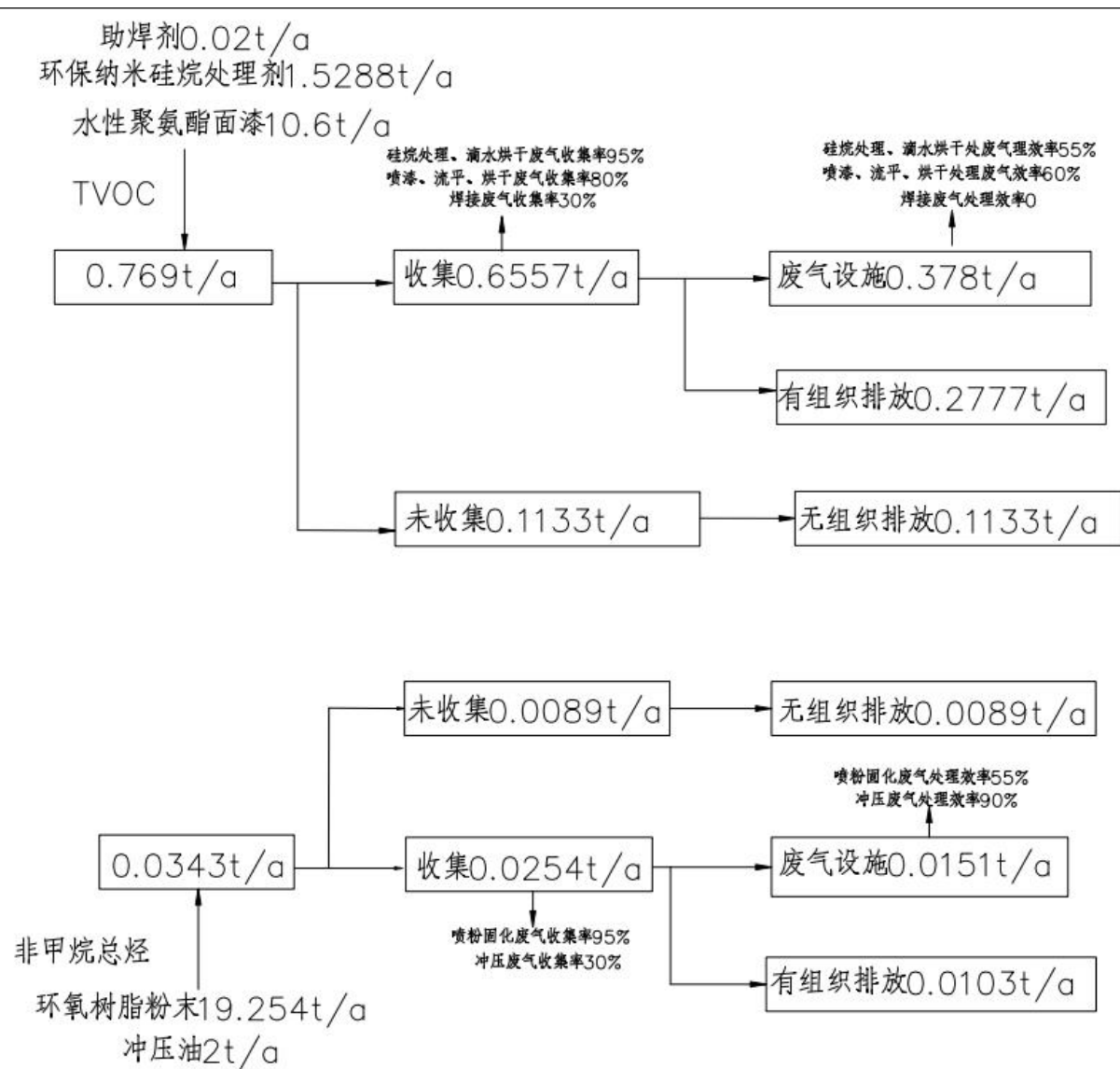
图 2-6 扩建后全厂 VOCs 平衡图
