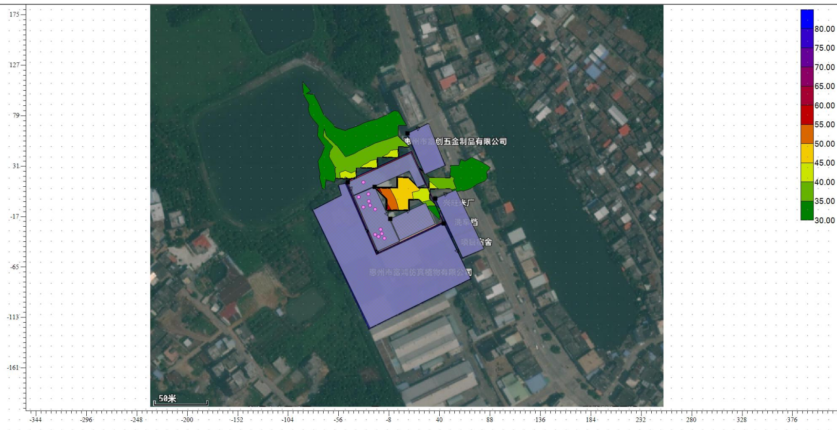
图 4-2 噪声预测图
