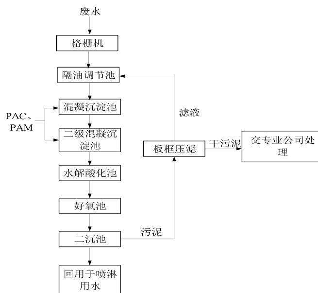
图 4-1 废水处理工艺流程图
