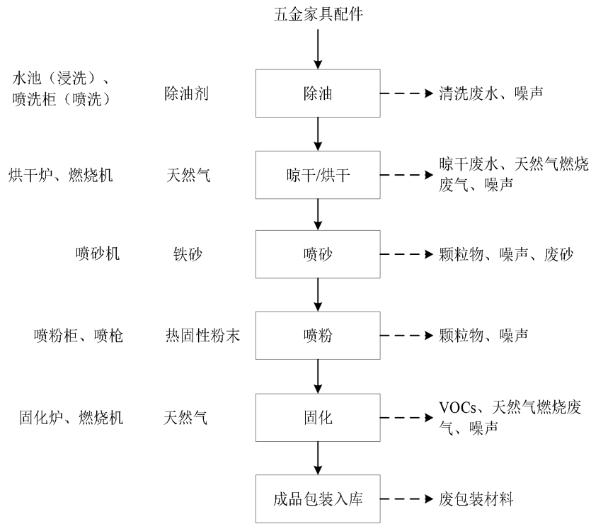
图2-2 五金家具配件生产工艺流程图
