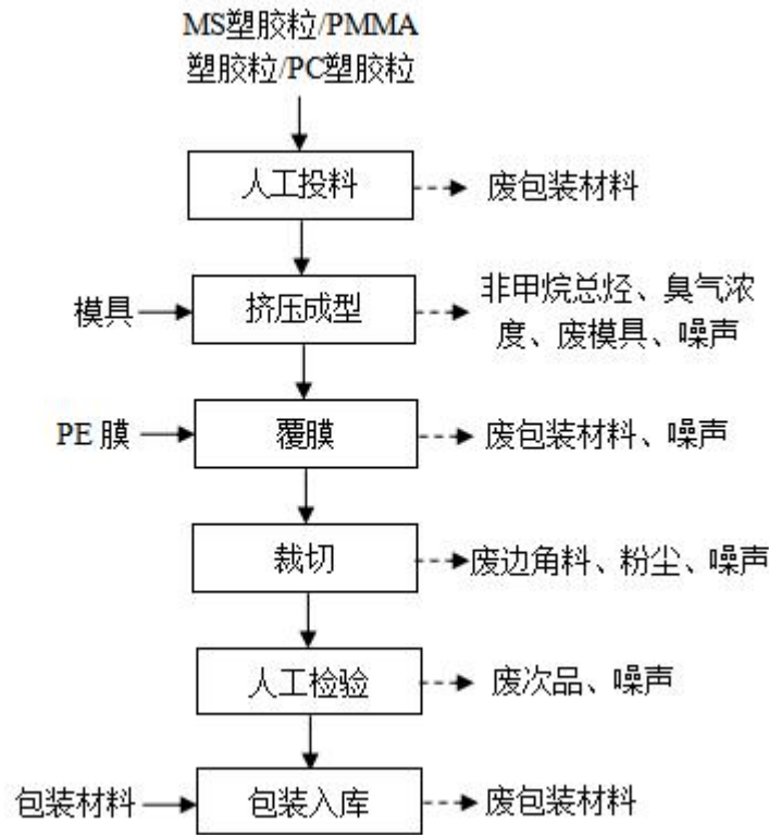
图 2-2 项目生产工艺流程及产污环节图
