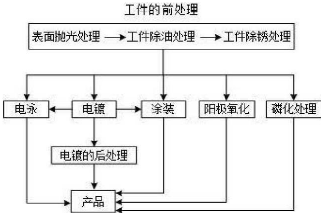
图 3.3-12 基地内企业基本生产流程图
