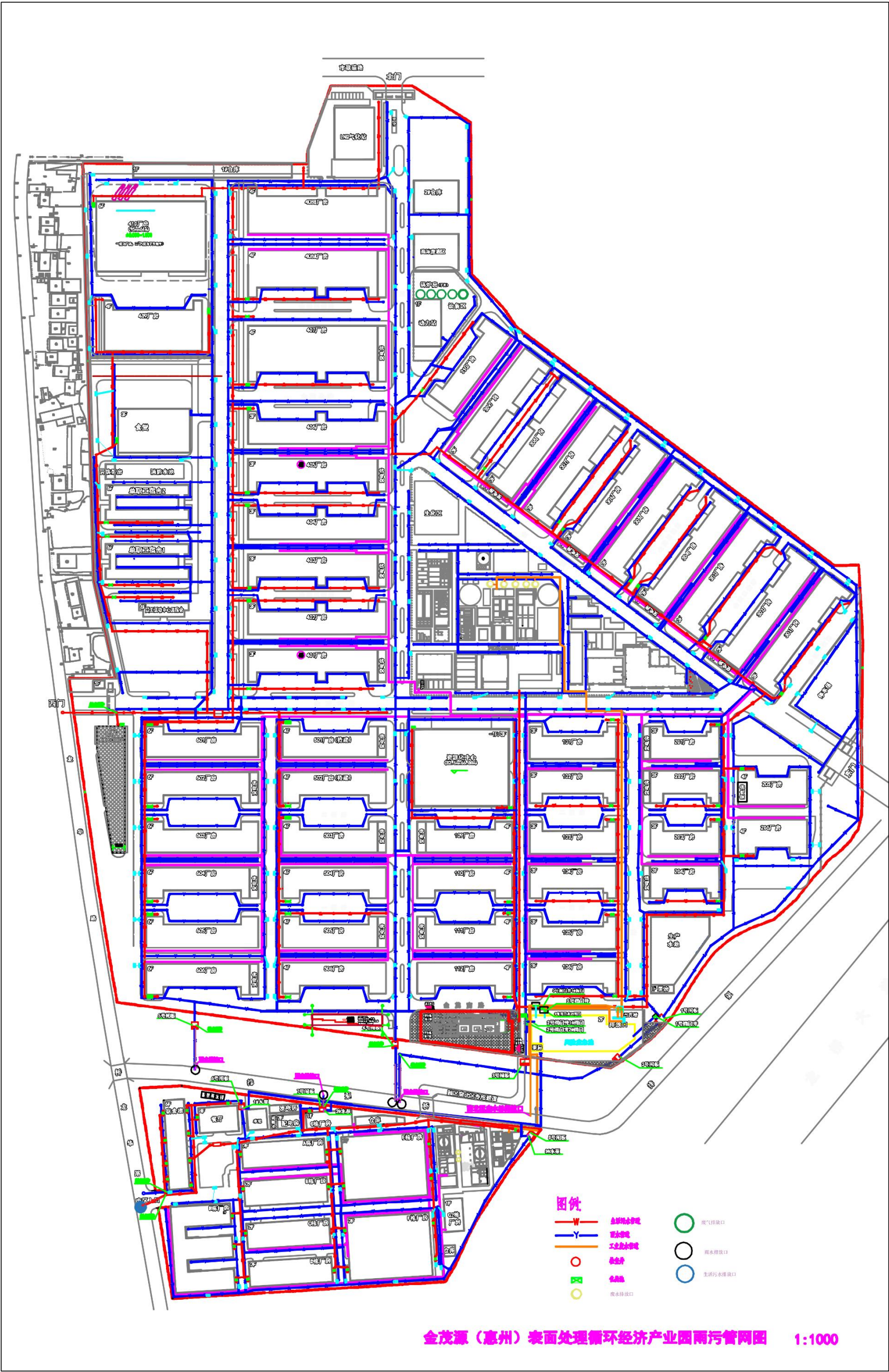
图 2.7-1 企业雨污管网图
