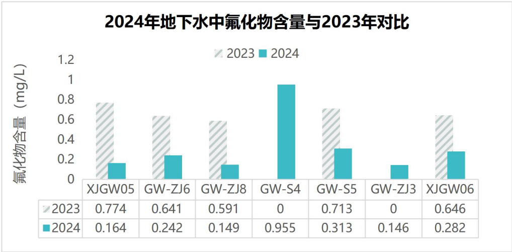
图 8.2-3 2024 年地下水中氟化物含量与 2023 年对比
