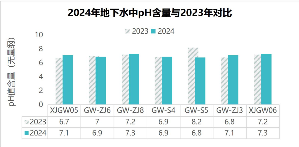
图 8.2-1 2024 年地下水中 pH 与 2023 年对比
