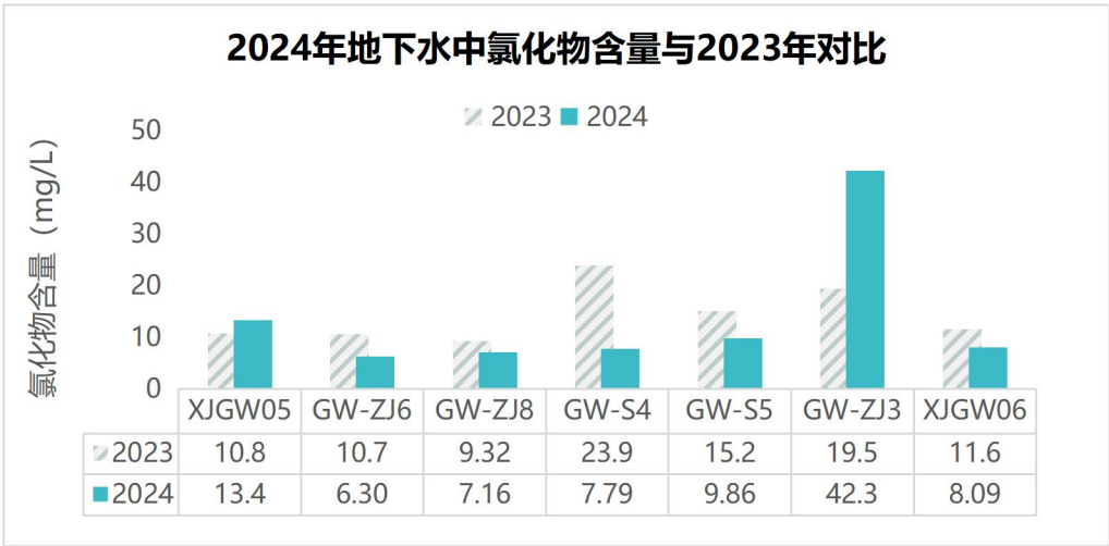
图 8.2-4 2024 年地下水中氯离子含量与 2023 年对比
