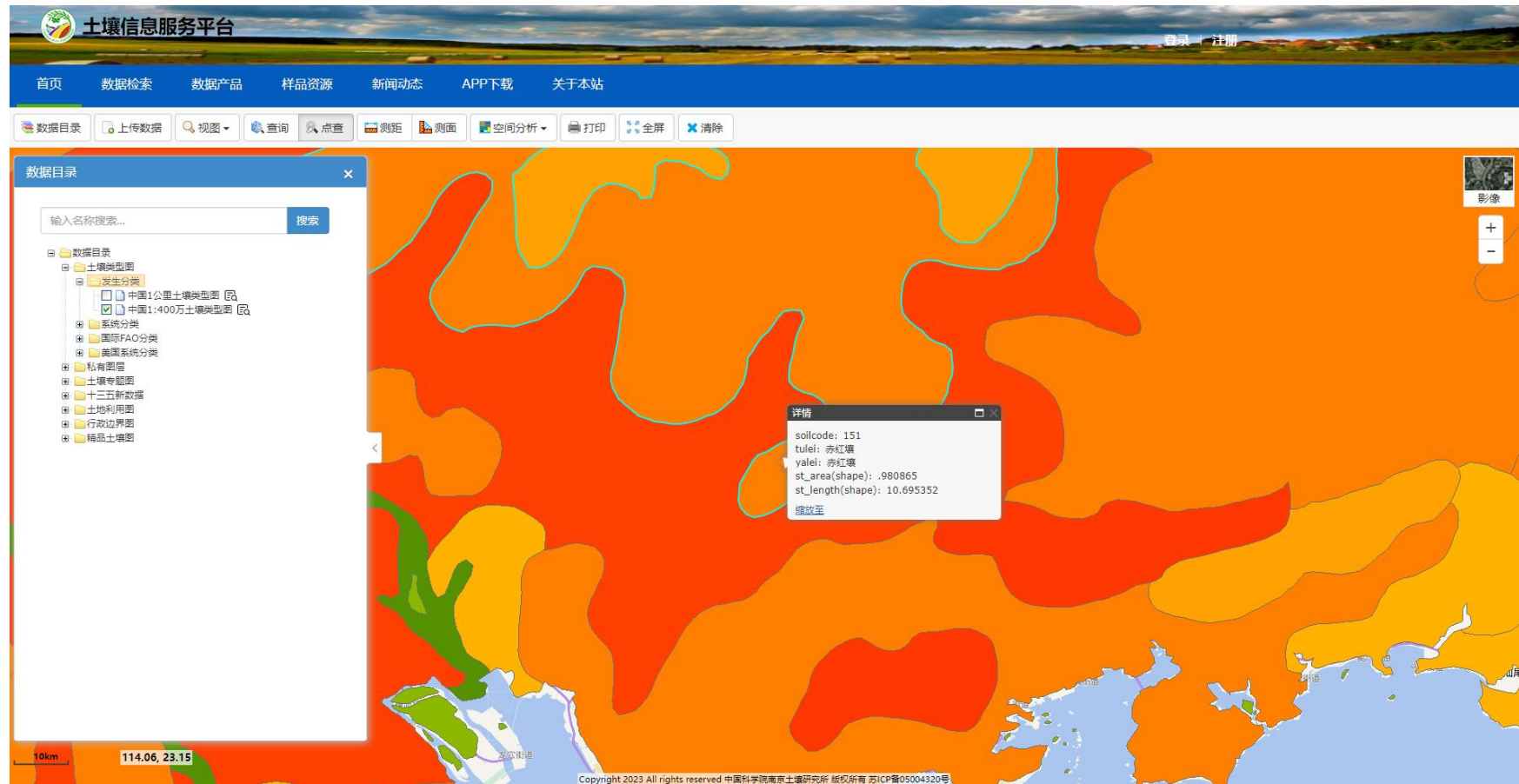
图 2.4- 1 项目所在地土壤类型图（图件来源国家土壤信息平台 1： 400 万土壤类型图）
