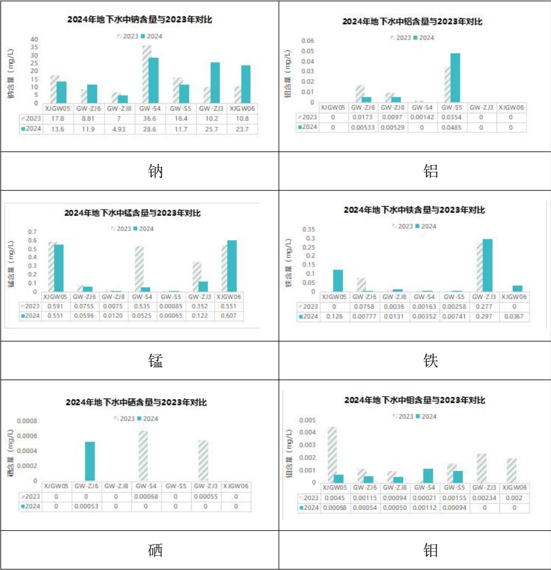
图 8.2-8 2024 年地下水中常规金属指标与 2023 年对比
