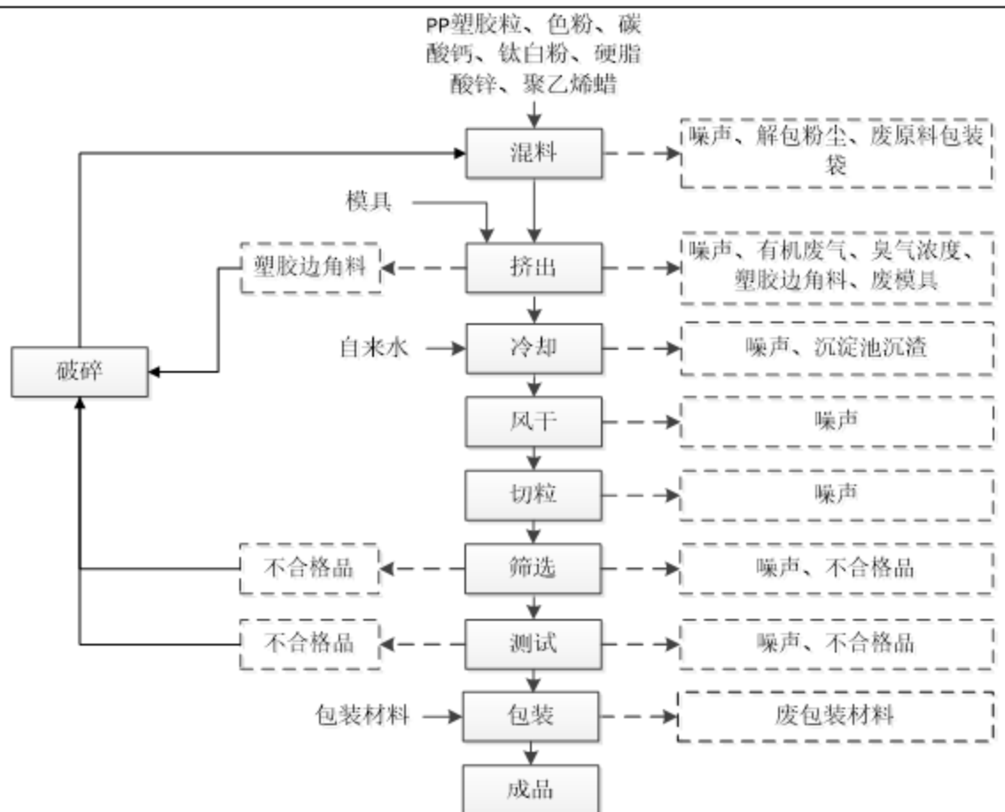
图 2-2 项目色母粒工艺流程及产污环节图
