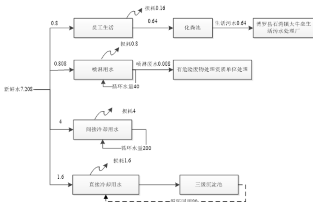
图 2-1 项目水平衡分析图（单位：m³/d）
