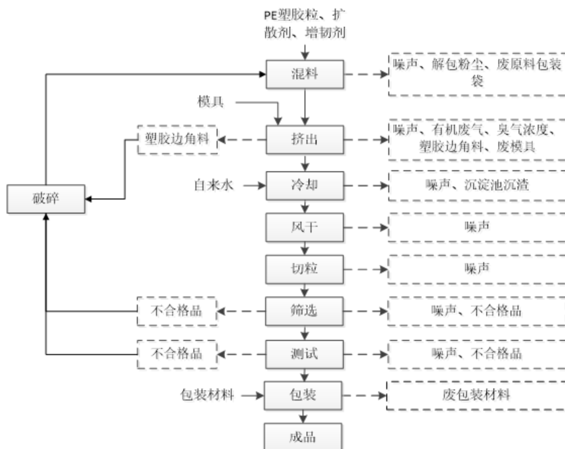
图 2-3 项目改性塑胶粒工艺流程及产污环节图
