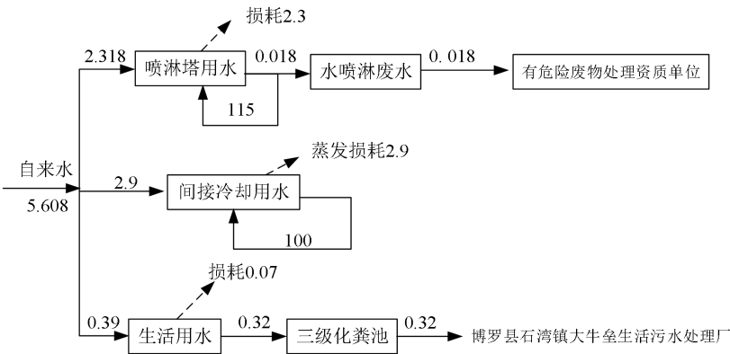
图 1 项目水平衡图 单位: t/d
