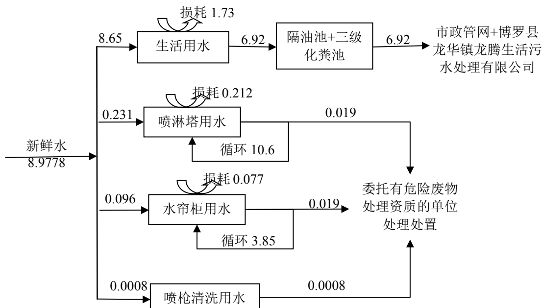
图 2-2 原有项目水平衡图 (t/d)
