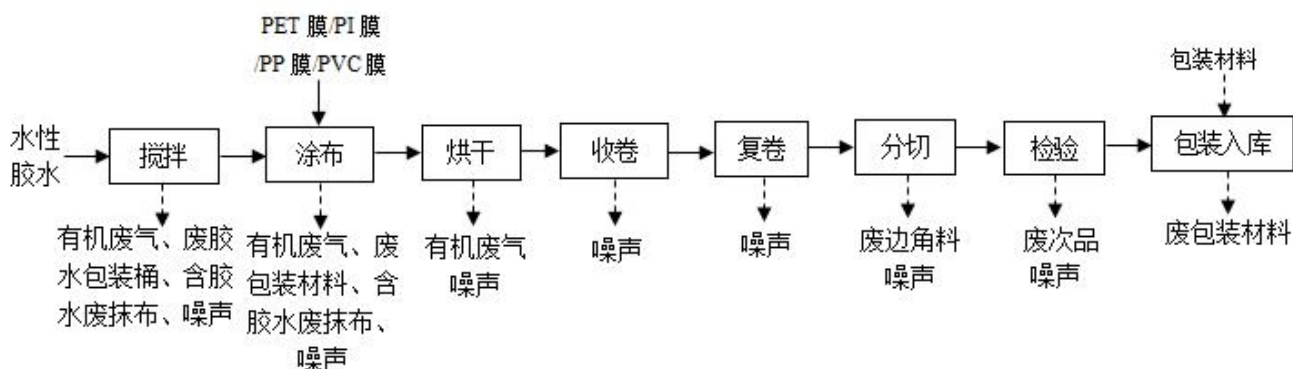
图 2-2 项目生产工艺流程及产污环节图
