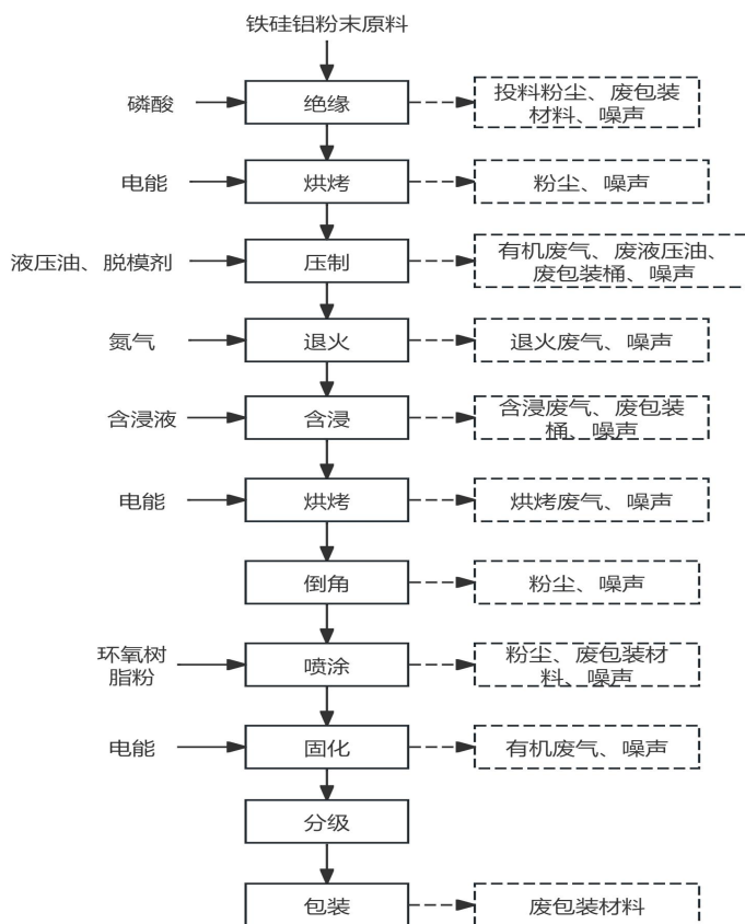
图2-2 软磁合金磁粉芯生产工艺流程图
